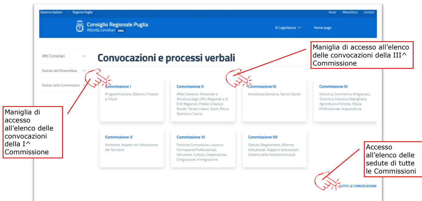
Fig. 18: Convocazione delle Commissioni – welcome page
